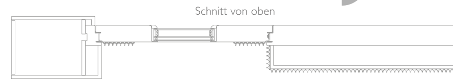
CHICAGO EDGEWATER mit Chicago-Verblendung RAL 8029 / ES s 204 / U b : 0,71
